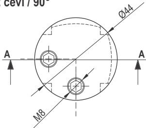
Konektor 2 cevi / 90°
