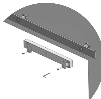
Montaža Soft Close usporivača vrata
