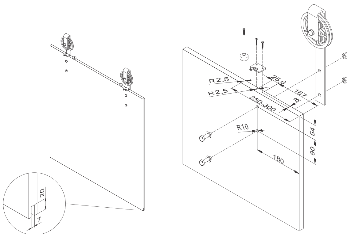
Montaža usmerivača pravca kretanja vrata
